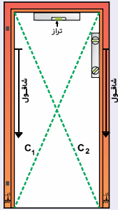
دو نخ شربری C1, C2 باید مساوی باشند و در نقطه تقاطع در تماس با یکدیگر باشند.
